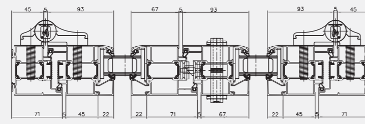
Coupe horizontale
