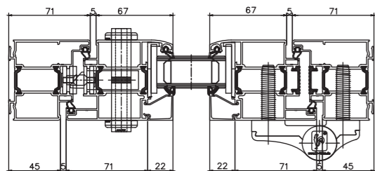
Coupe horizontale
